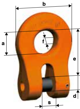
KRW Kuppelring
