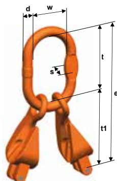
VMXKW 2 Kuppelaufhängegarnitur
