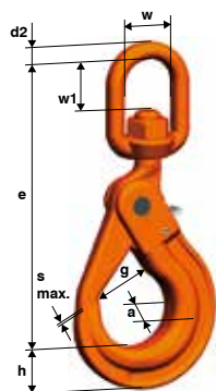
WLHBW Wirbelsicherheitslasthaken
