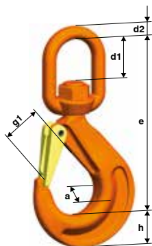
WSBW Wirbelhaken
