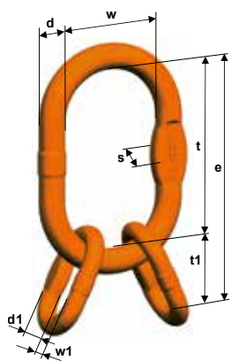
VW Vierstranggarnitur
