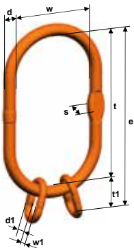
VSW 2/4 Übergroße Aufhängegarnitur
