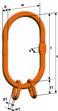
VLW 2/4 Aufhängegarnitur
