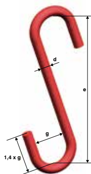
SM S-Haken
