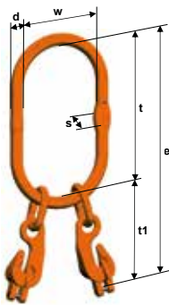
LXKW 2 Kuppelaufhängegarnitur
