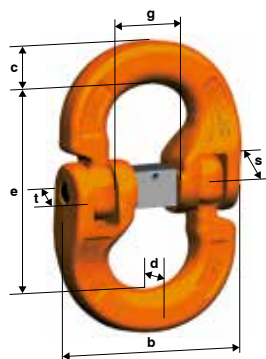
CLW Connex Verbindungsglied
