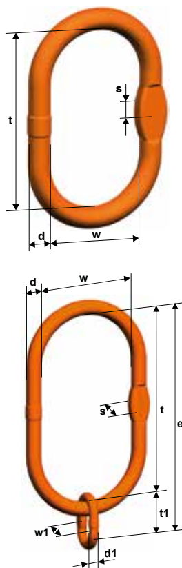
VSAW 1 Aufhängegarnitur
