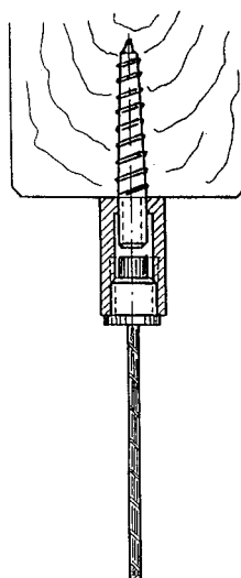
Befestigung mit Stockschrabe. Seil mit ASS Zylinderterminal verpresst
